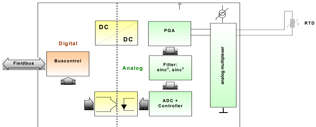
Abbildung 3: Blockdiagramm
