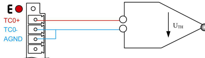
Abbildung 7: Thermoelement interner isothermer Block
