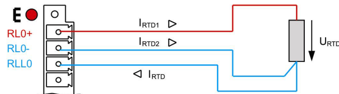
Abbildung 5: Dreileitertechnik
