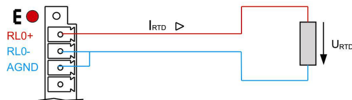
Abbildung 4: Zweileitertechnik
