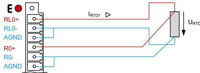
Abbildung 6: Vierleitertechnik
