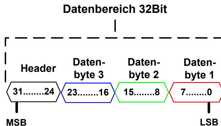
Abbildung 8: Datenbereich Temperaturmodul
