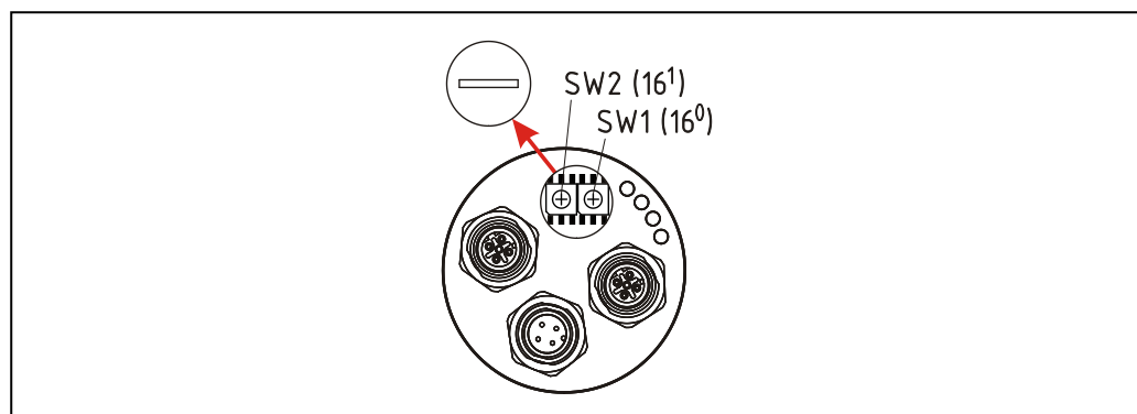
Abbildung 3: EtherNet/IP™ Node-Adresse, Schalterzuordnung
