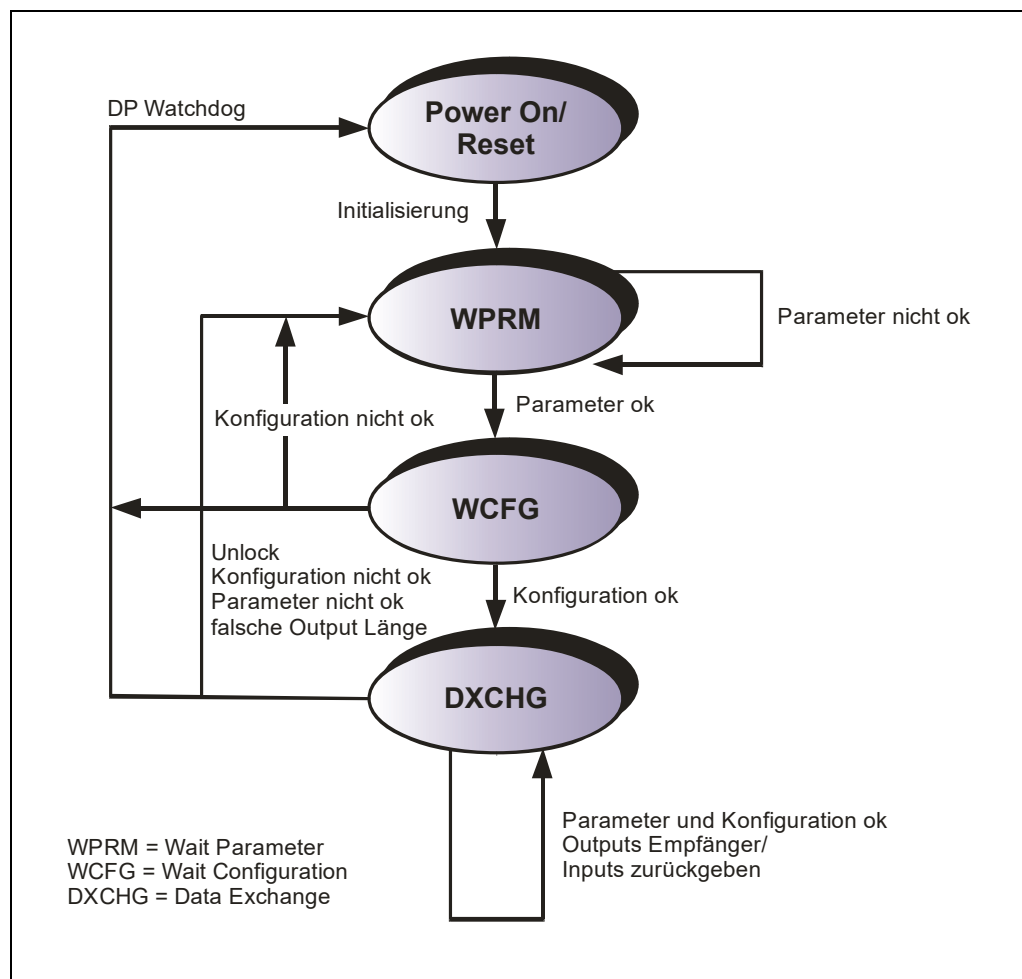
Abbildung 4: DP-Slave Initialisierung
