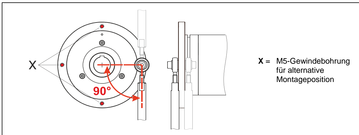
Abbildung 9: Gelenkkopfstab – Montagevarianten
