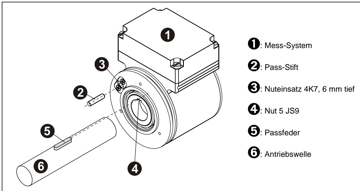
Abbildung 5: Formschluss
