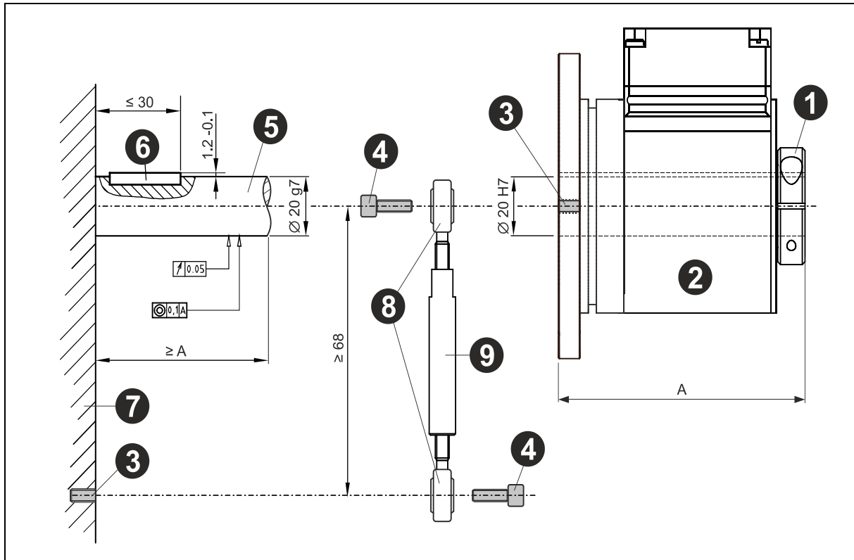
Abbildung 8: Anforderungen an die Wellenaufnahme
