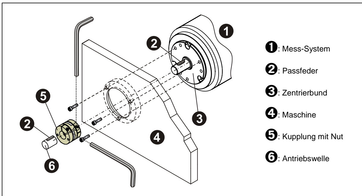
Abbildung 2: Flansch-Montage
