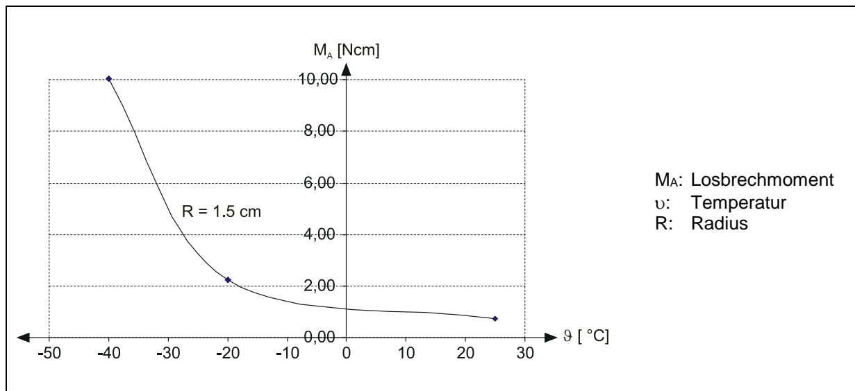
Abbildung 3: Losbrechmoment
